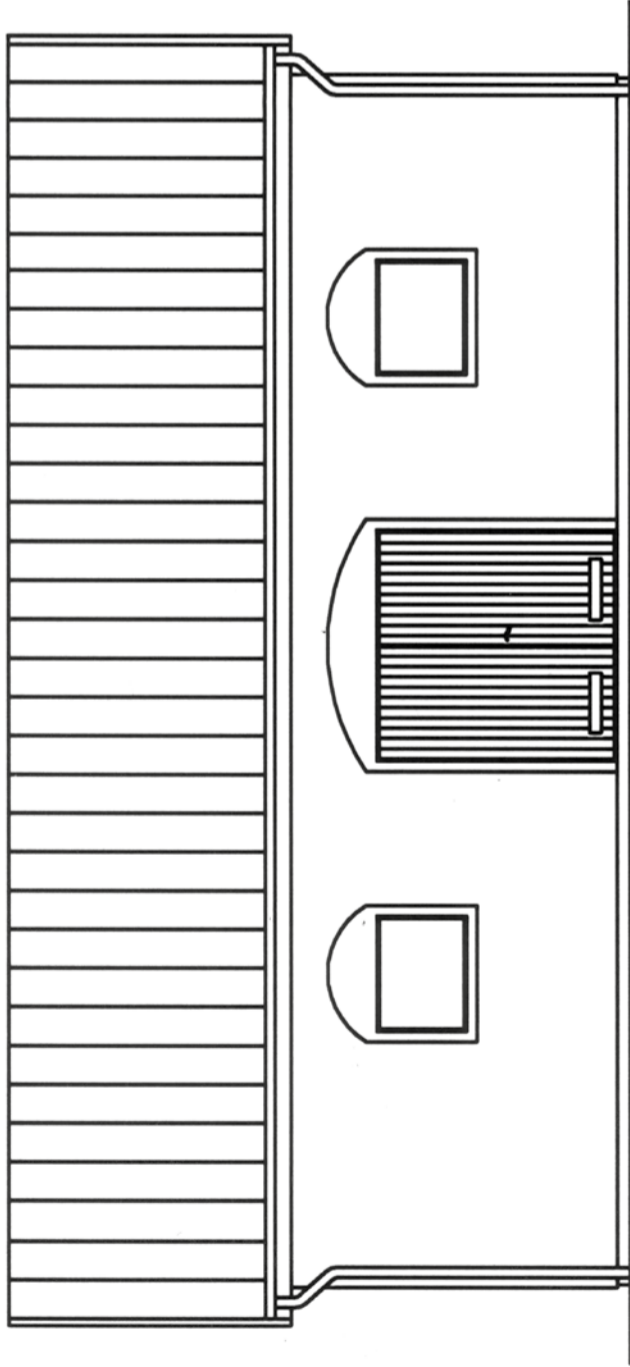
LÅNGFASAD ENTRÉ
